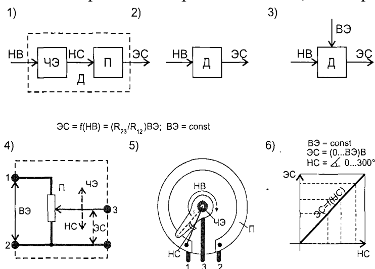
Рисунок 2.2 - Моделі датчиків
