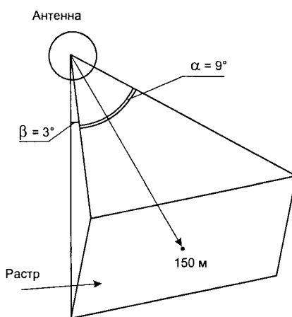
Рисунок 2.31 Растр Радівипромінювача
