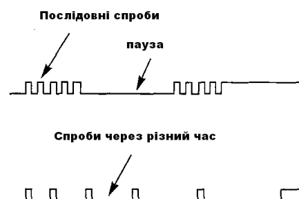
Рисунок 6.22 - Алгоритми перезавантаження шини CAN
