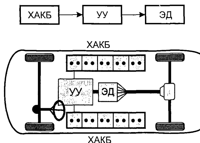
Рисунок 10.1 - Класична схема електромобіля:
