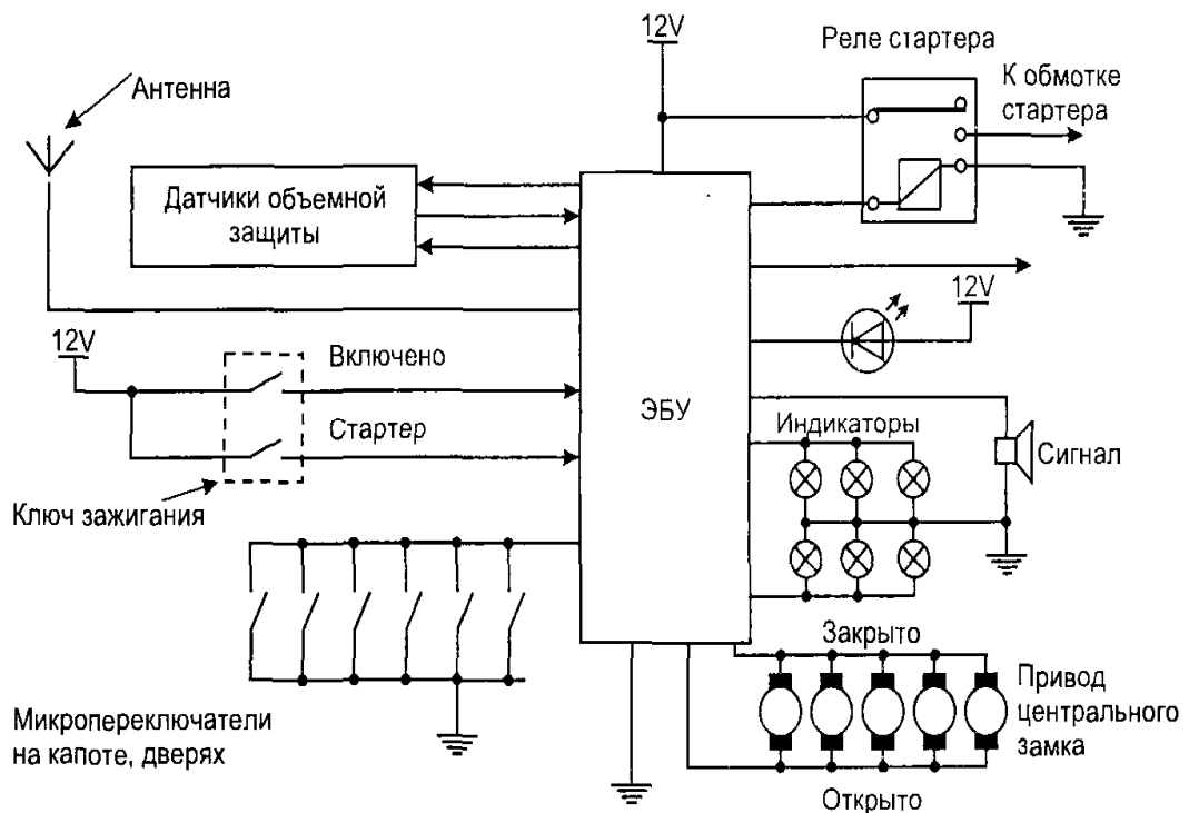
Рисунок 5.36 - Блок-схема базової антивикрадацької системи
