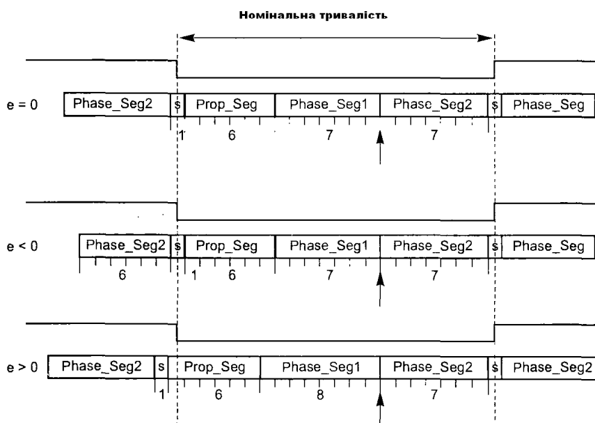
Рисунок 7.6 - Синхронізація передачі біта
